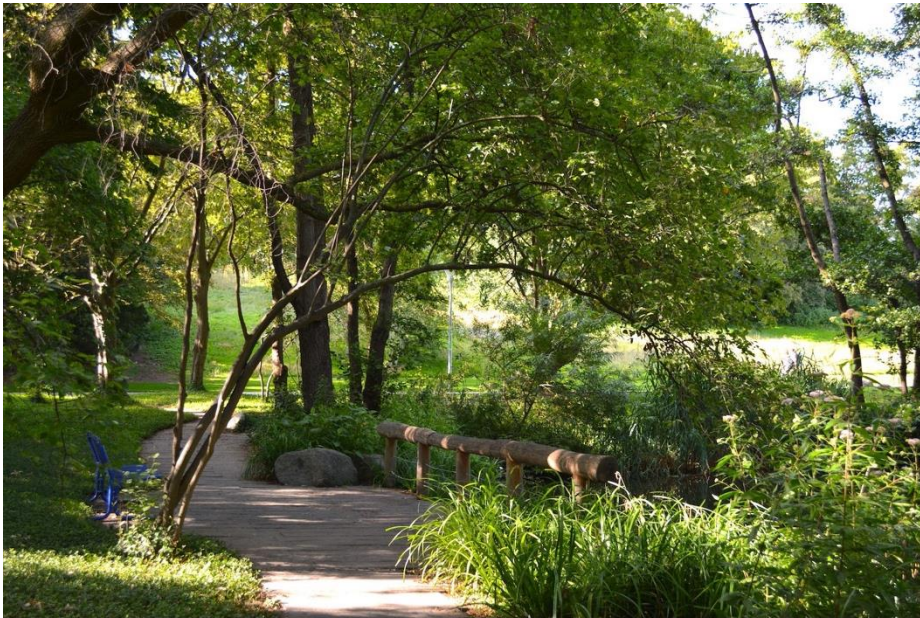
Abbildung 5: Gebirgsbach
